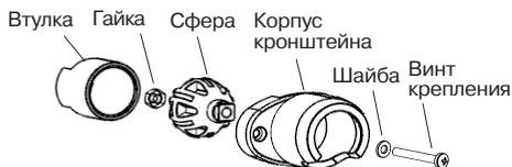
Рисунок 1 – Детали кронштейна
